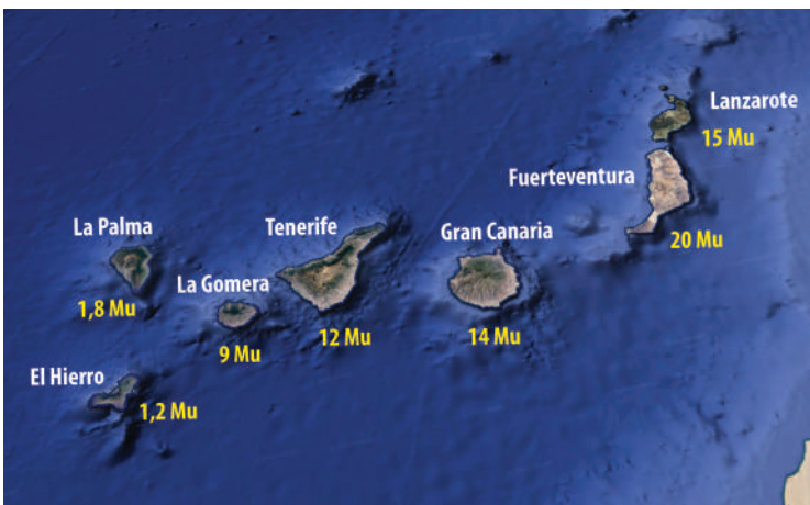
Irla bakoitzeko arroka zaharrenak aztertuta, argi ikus daiteke Kanarietako bolkanismoa mendebalderantz mugitzen dela. GOOGLE EARTH MOLDATUTA
