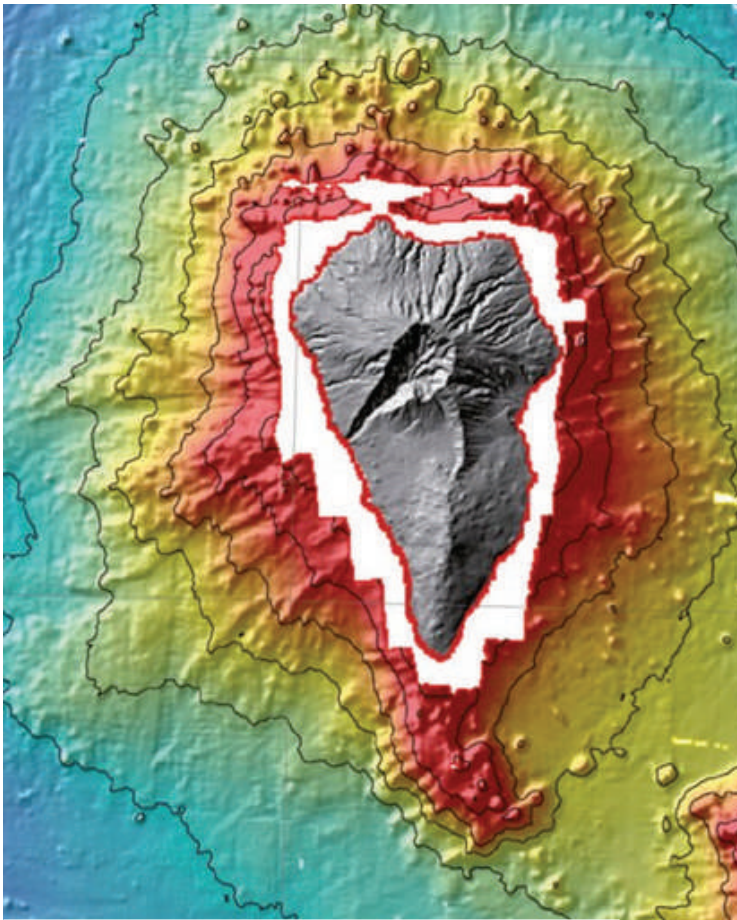
La Palmako eraikin bolkanikoaren benetako forma eta tamaina. IEO
