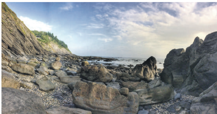
Kardalako labarretako flysch beltza. GONZALO TORRE
