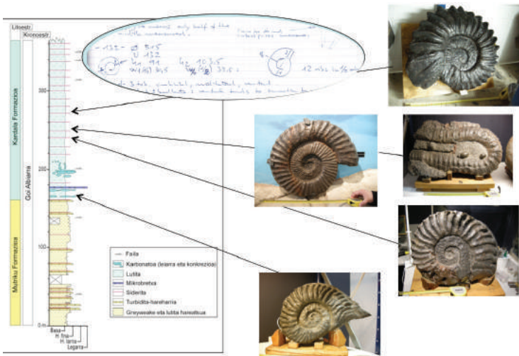
Zutabe estratigrafikoa eta amoniteen kokapena.
